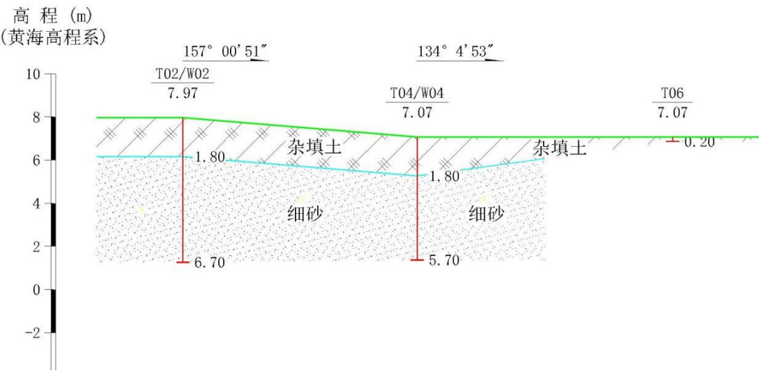
图 3-4 典型剖面图
