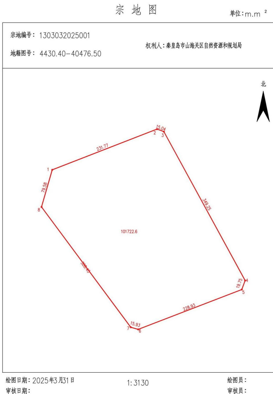
图 2-2 地块宗地图
