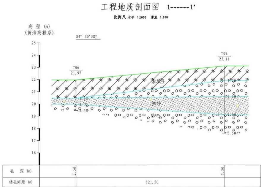
图 3-6 1-1' 线剖面图
