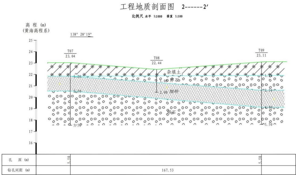
图 3-7 2-2' 线剖面图
