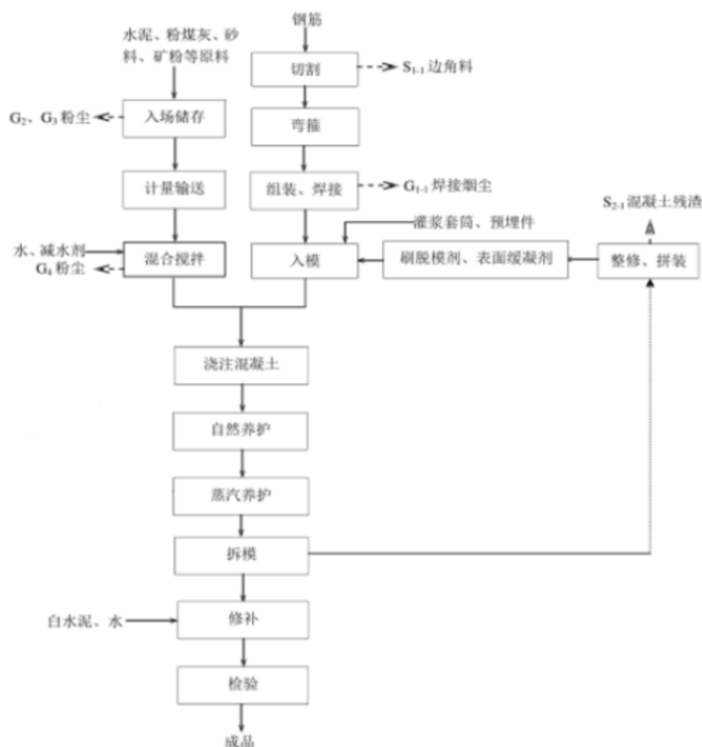
图 4.4-3 PC 构件工艺流程图
