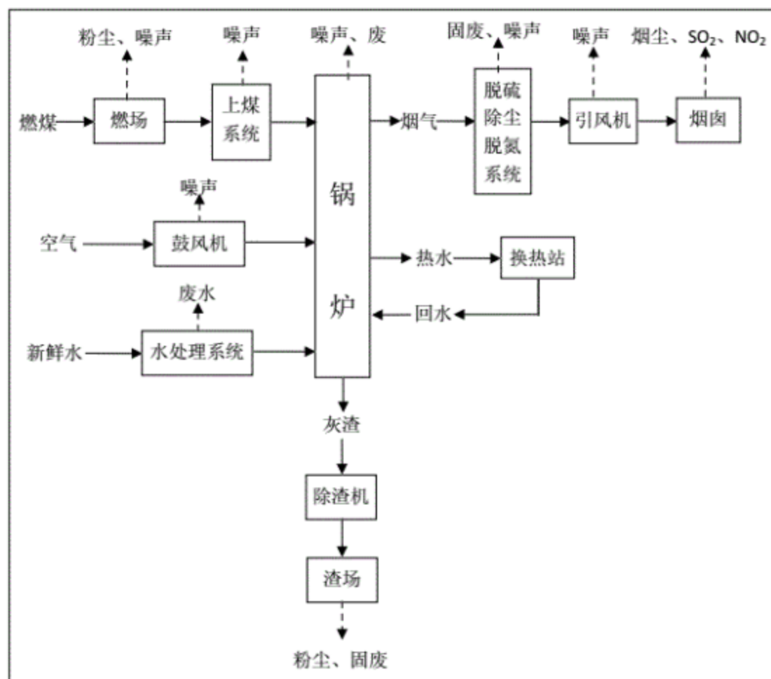
图 4.4-3 富阳热力生产工艺流程图
