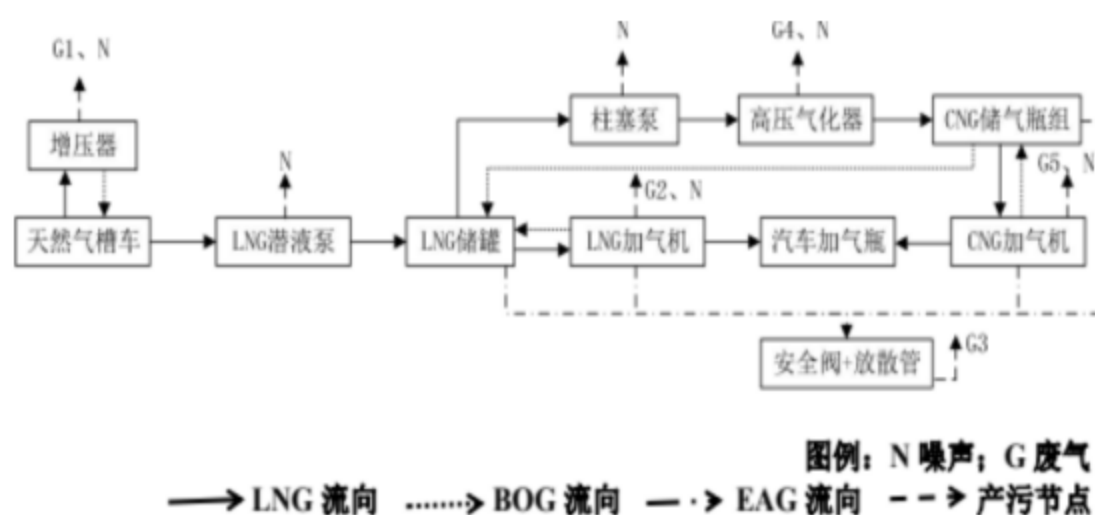
图 4.4-2 华润燃气生产工艺流程图
