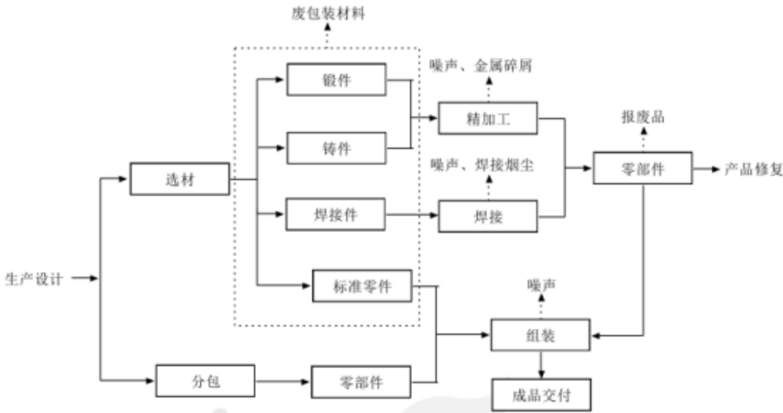
图 4.4-4 企业生产流程图
