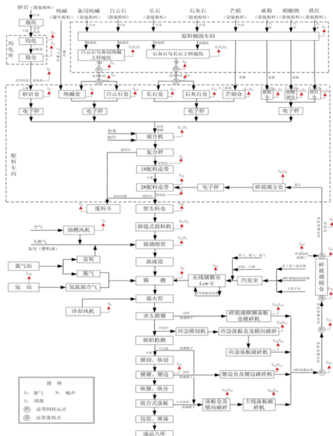
图 4.4-1 耀华玻璃生产工艺流程图
