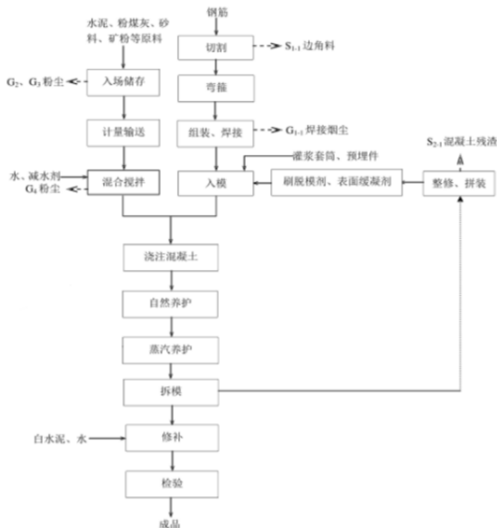
图 4.4-3 PC 构件工艺流程图
