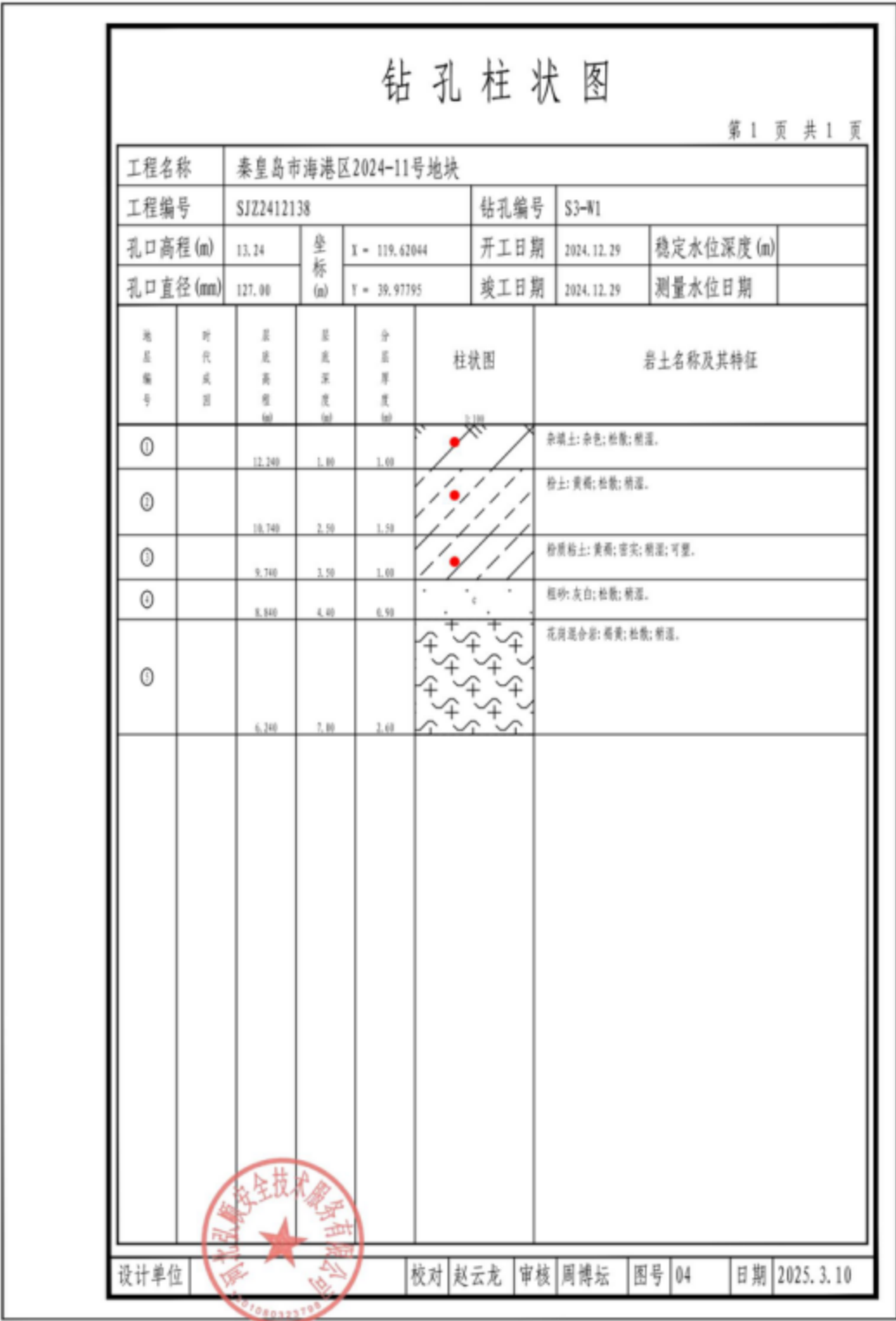
图 3.1-7 钻孔柱状图
