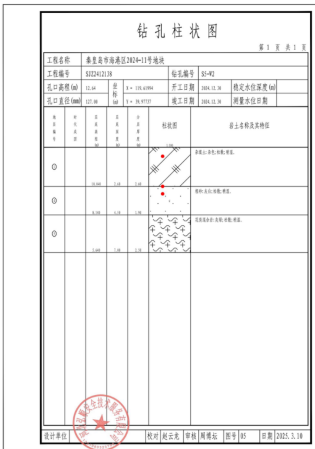
图 3.1-8 钻孔柱状图
